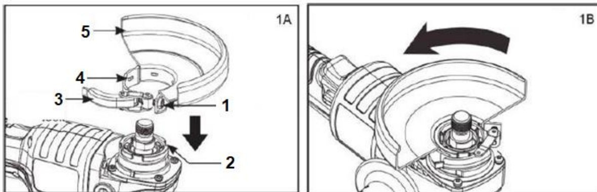
1. Skrutka 2. Zárezy 3. Upínací zámok 4. Vydutia 5. Kryt
